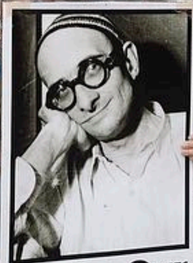
Radu Gyr
